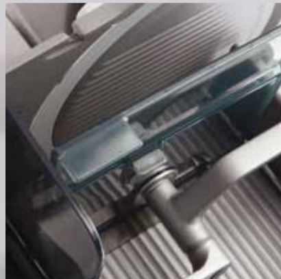
Resthalter mit Magnethalterung Remnant holder with magnetic bracket
